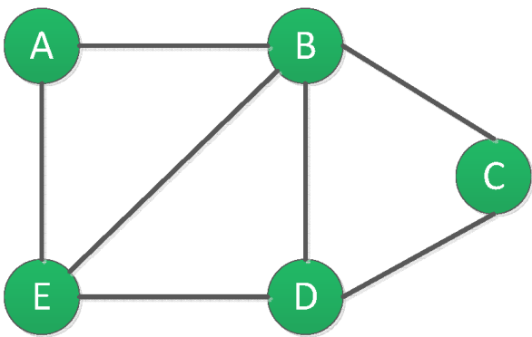
A. 无向图
