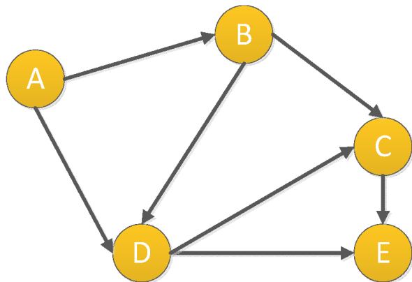
B. 有向图
